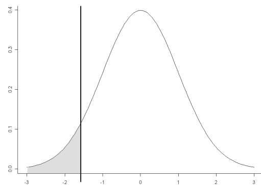
図2. 片側検定 (対立仮説が \mu < \mu_0 のとき)
