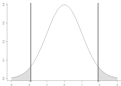
図1. 両側検定 (対立仮説が \mu \neq \mu_0 のとき)
